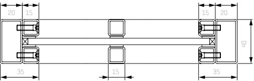
Horizontalschnitt 1-flüglige Retro Loft Schiebetür
