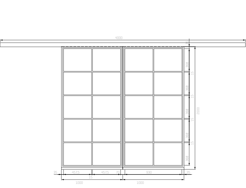
2-flüglige Stahl-Lofttür
