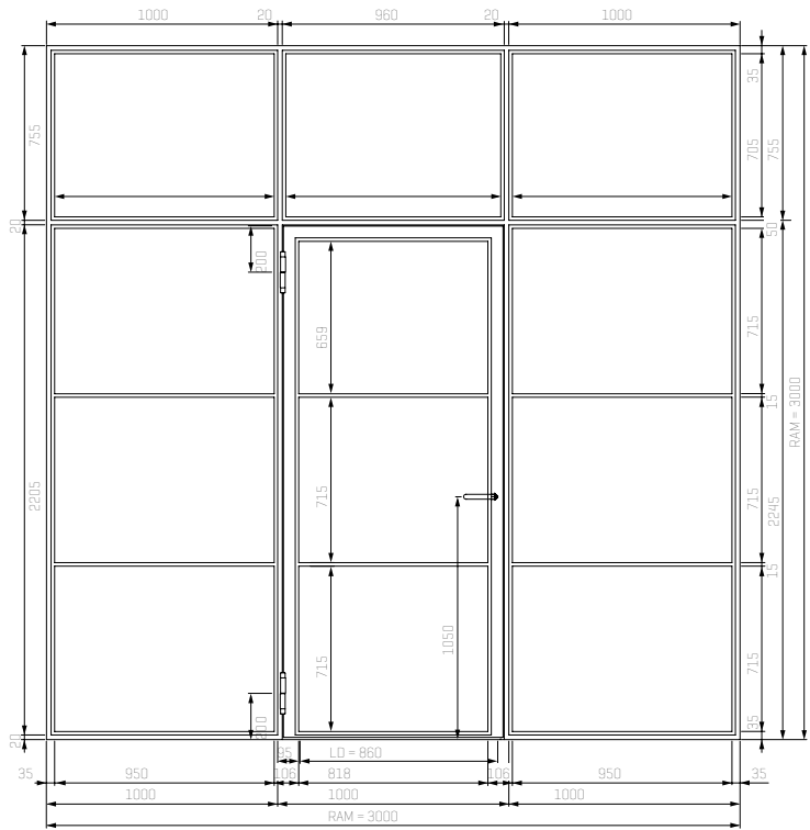
1-flüglige Stahl-Lofttür mit Seitenteilen und Oberlicht
