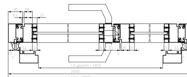
Horizontalschnitt 2-flüglige Stahl-Lofttür
