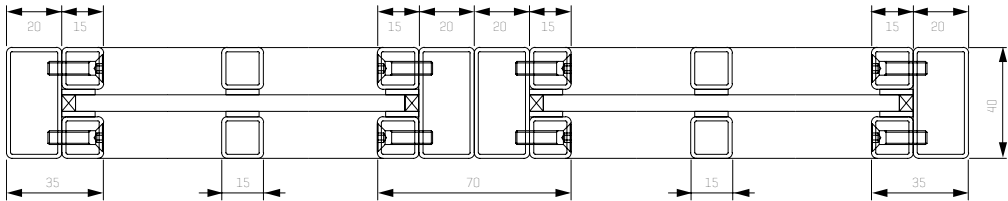
Horizontalschnitt 2-flüglige Retro Loft Schiebetür
