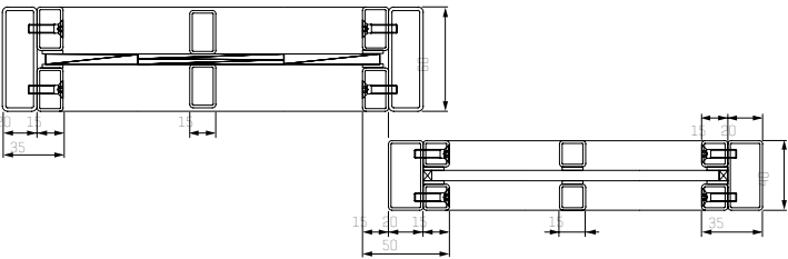
Horizontalschnitt 2-flüglige Stahl-Lofttür
