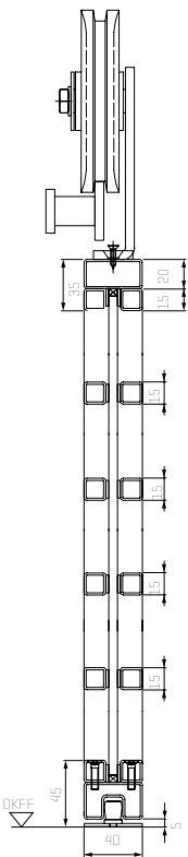
Vertikalschnitt 2-flüglige Retro Loft Schiebetür
