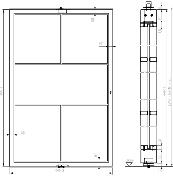
Pivottür in Standardausführung mit 50 mm breitem Rahmenprofil und 50 mm hohem Sockel, Motiv 2
