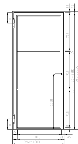
1-flüglige Stahl-Lofttür
