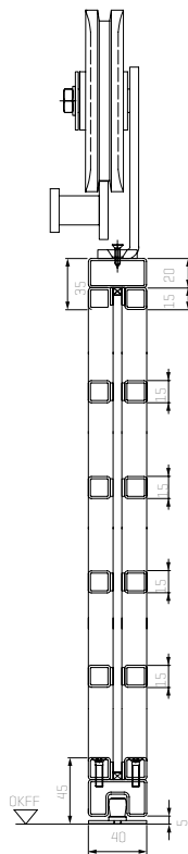
Vertikalschnitt 1-flüglige Retro Loft Schiebetür
