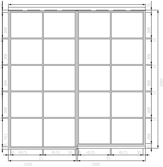
2-flüglige Stahl-Lofttür
