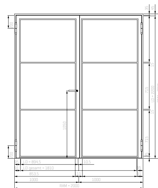
2-flüglige Stahl-Lofttür
