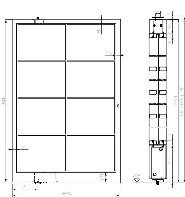
Pivottür mit 50 mm breitem Rahmenprofil und 120 mm hohem Sockel, symmetrische Sprossenaufteilung
