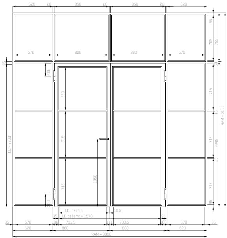
2-flüglige Stahl-Lofttür mit Seitenteilen und Oberlicht
