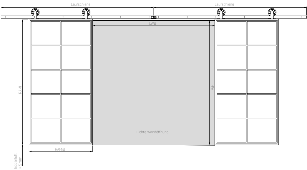
2-flüglige Retro Loft Schiebetür
