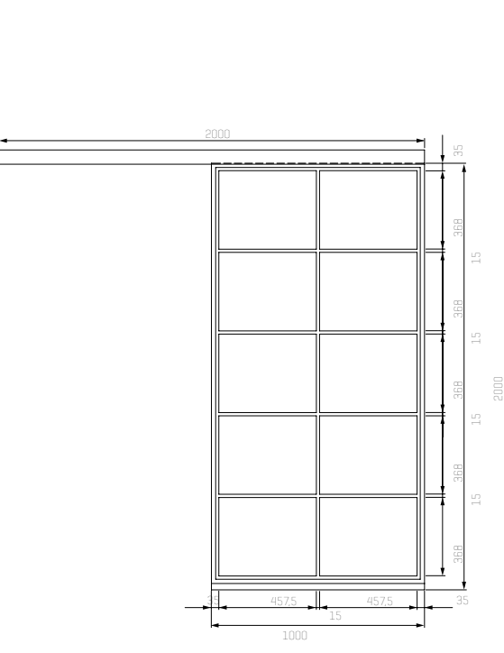
1-flüglige Stahl-Lofttür
