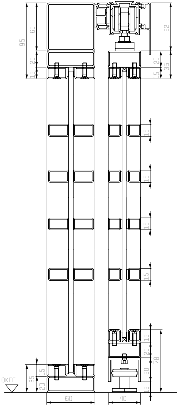
Vertikalschnitt 2-flüglige Stahl-Lofttür
